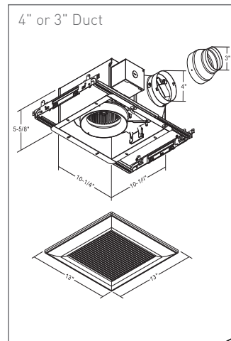
FV-0511VFC1
