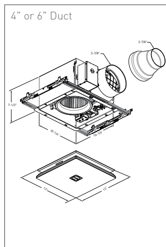
FV-0511VKSL3K
