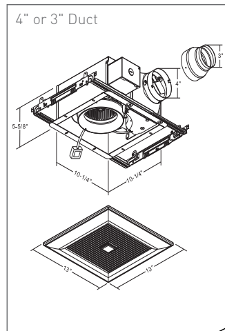
FV-0511VF1
